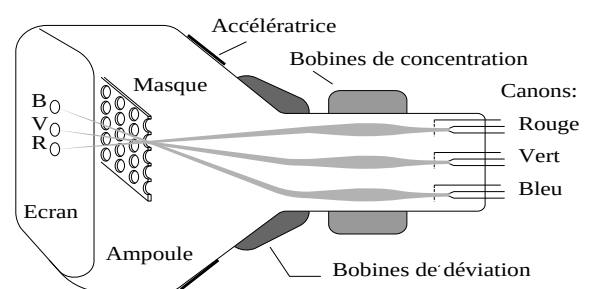
Fig. 5-4 : Ecran cathodique couleur.
